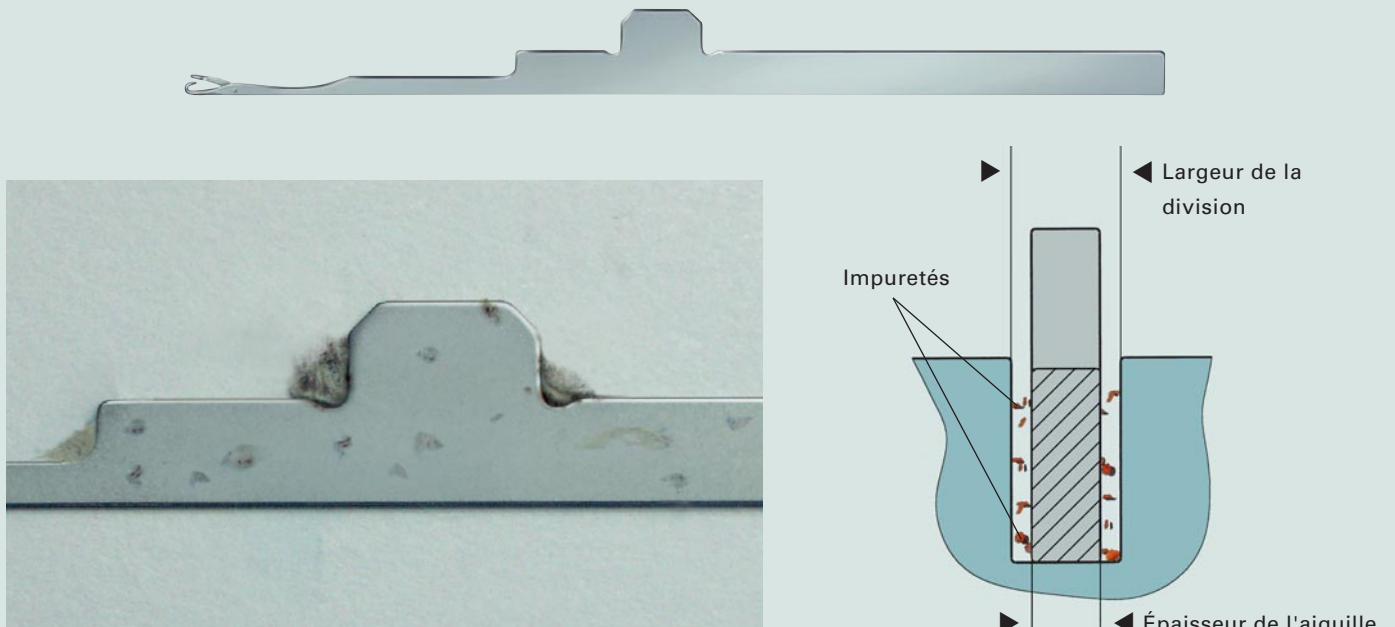
COUPE: AIGUILLE DANS SA DIVISION
